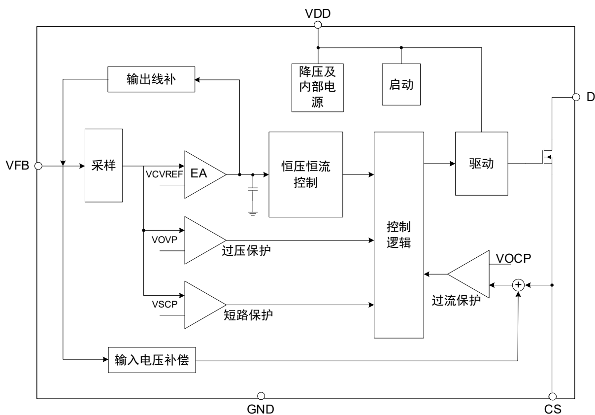
图 2 CM1713 功能模块框图
