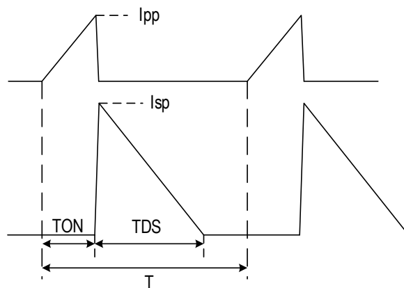
图 5 恒流工作原理图
