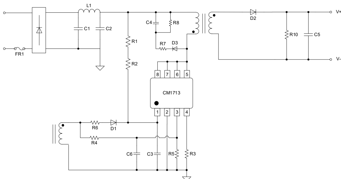
图 1 CM1713 典型应用电路
