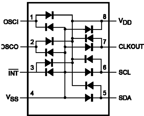
管脚二极管保护图：
