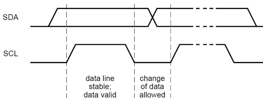
I 2 C总线上的位传送
