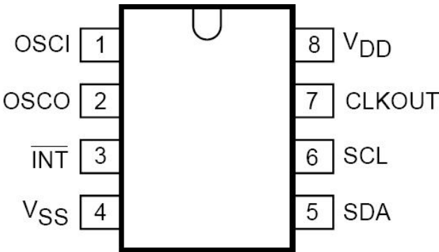
D8563(DIP8/SOP8/MSOP8/TSSOP8/DFN8)
