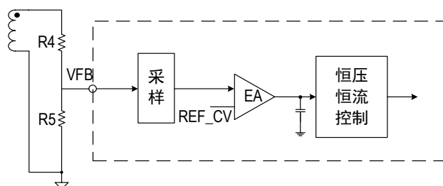
图 4 恒压工作原理图
