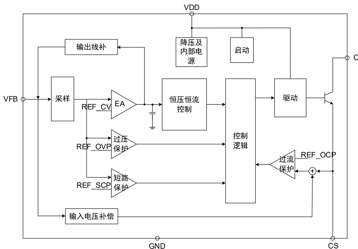
图 2 CM1702 功能模块框图
