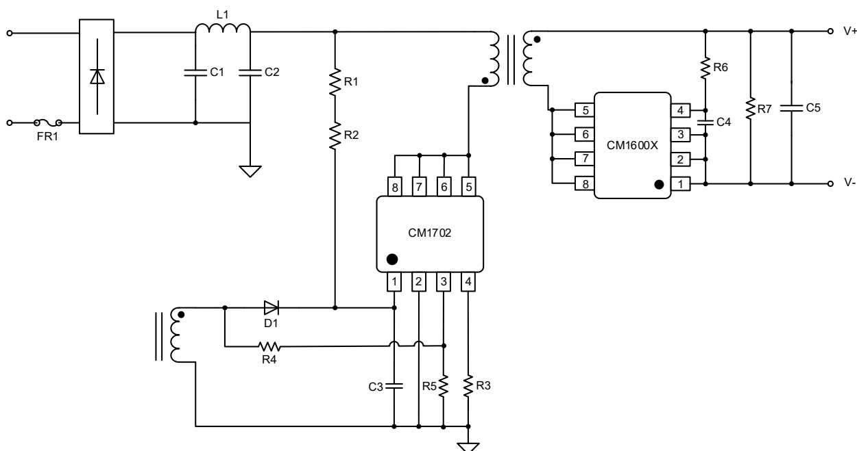
图 1 CM1702 典型应用电路
