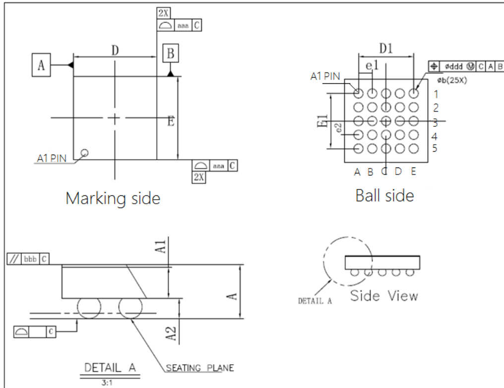
图 22 WLCSP25(2.410 x 2.415 mm)封装框图
