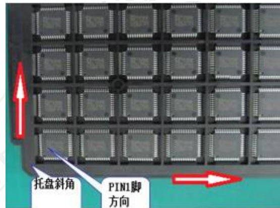
图 24 PIN1 位置示意
