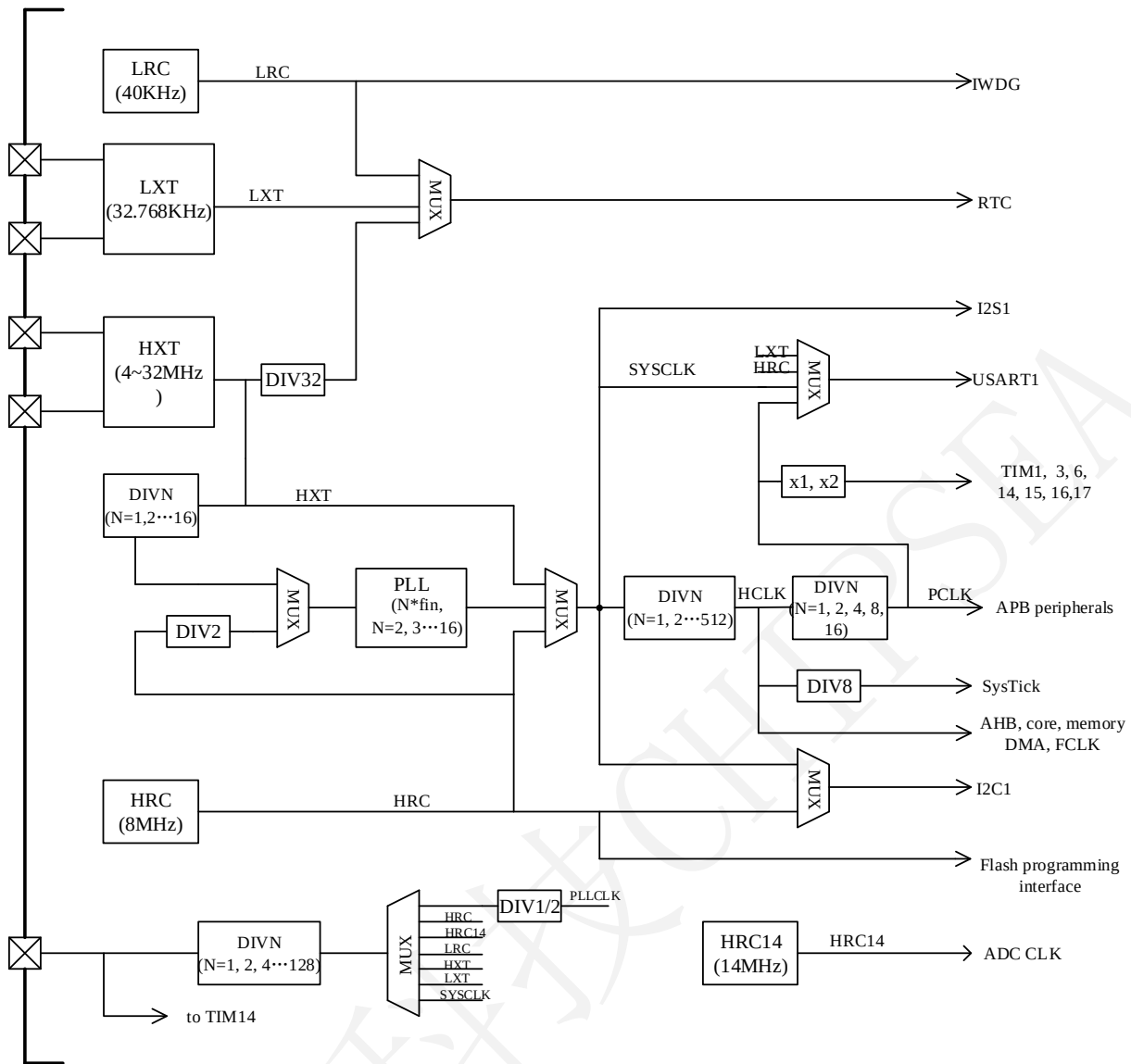
图 10 芯片时钟树
