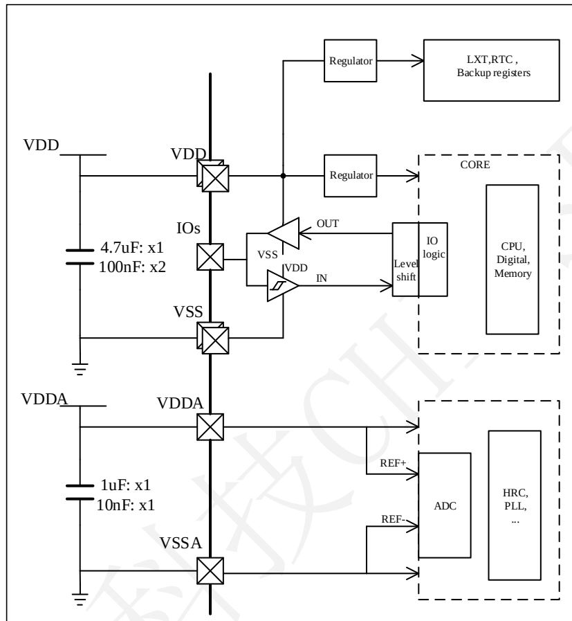
图 11 电源方案
