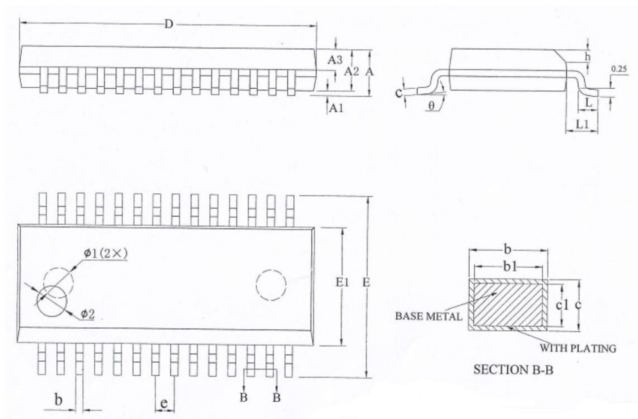
图 22 SSOP28 封装框图
