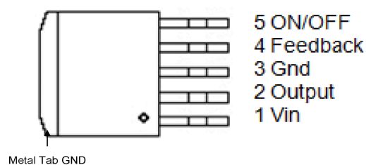
TO- 252-5
