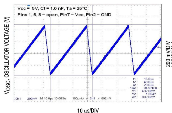
振荡器定时电容波形
