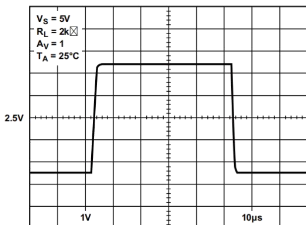
图 29.大信号瞬态响应
