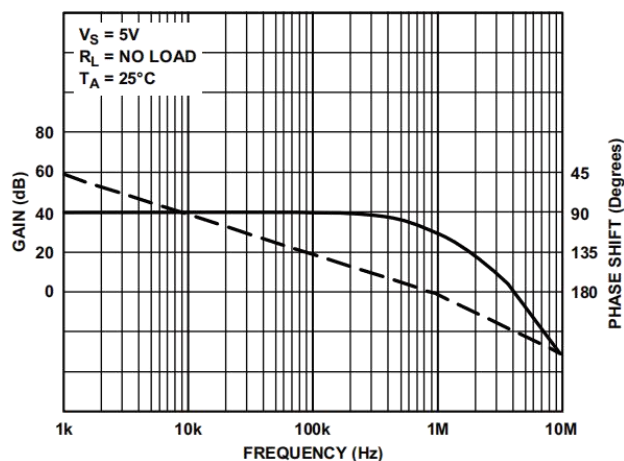
图 30.开环增益和响应与频率的关系
