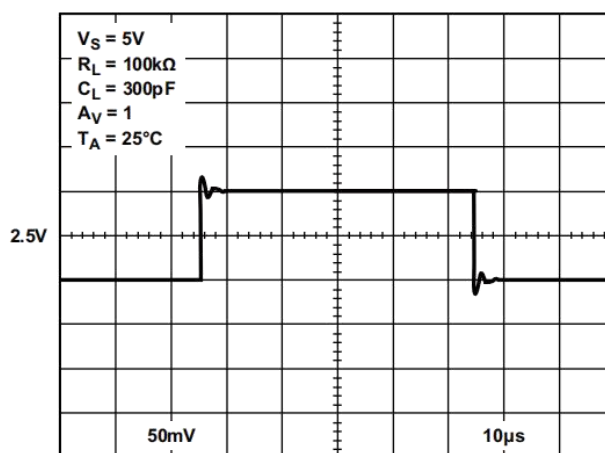
图 28.小信号瞬态响应
