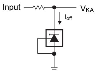
图 22 关断器的测试电路
