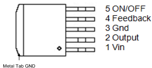
TO- 252-5
