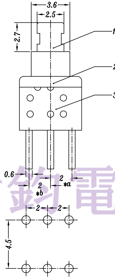
P.C.B. LAYOUT
