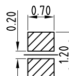
METAL MASK T=0.10 TOLERANCE±0.05(钢网推荐图)
