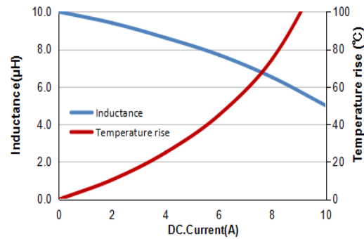
FSA0650-100MT
