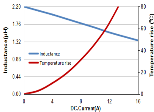
FSA0650-2R2MT
