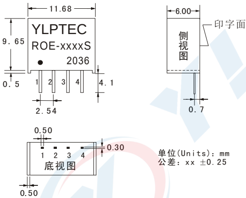
1) 外观尺寸
