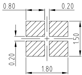
METAL MASK T=0.10 TOLERANCE±0.05(钢网推荐图)
