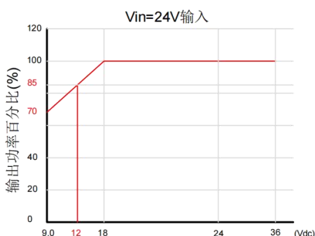
电压降额曲线
