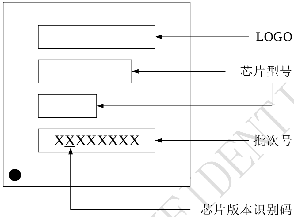
图 5-4 丝印说明图
