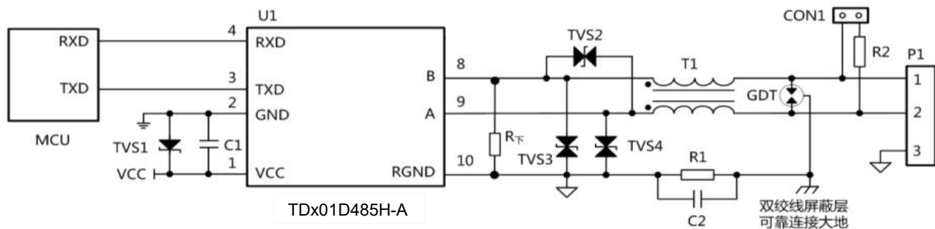
图 3. EMC 推荐电路
