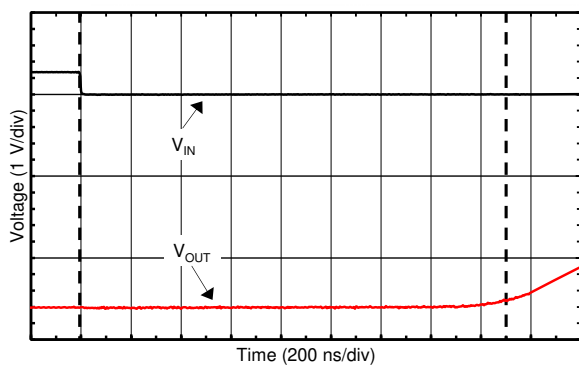
图 6-27. No Phase Reversal
