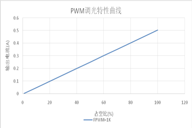
DIM 脚 PWM调光特性曲线
