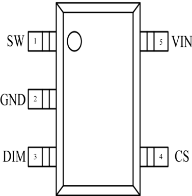
SOT23-5
