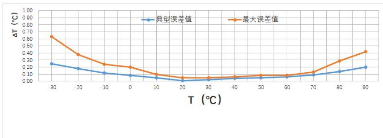
图 7- 3 M601W/M1601W/M1820W 精度误差曲线
