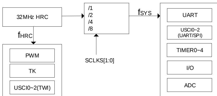
SC95F861X 内部时钟关系
