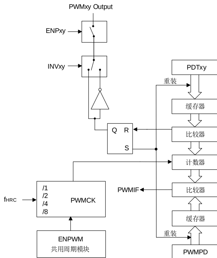
SC95F861X PWM 独立模式框图
