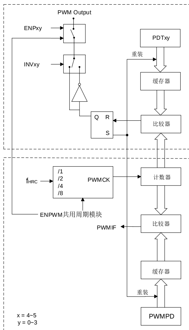
SC95F861X PWM 结构框图
