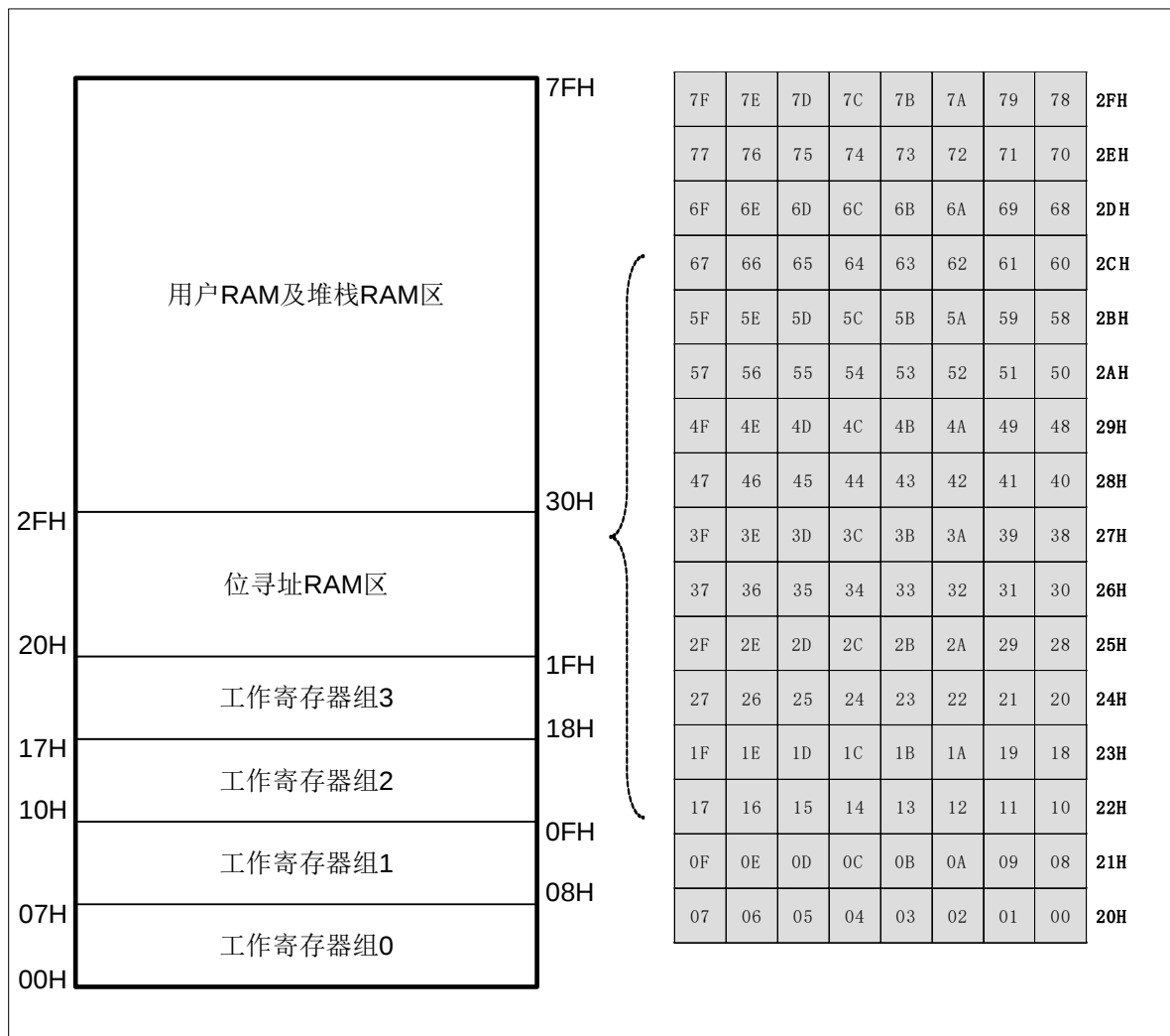
SRAM 结构图
