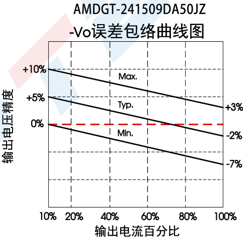
图 9 (辅路误差包络曲线)
