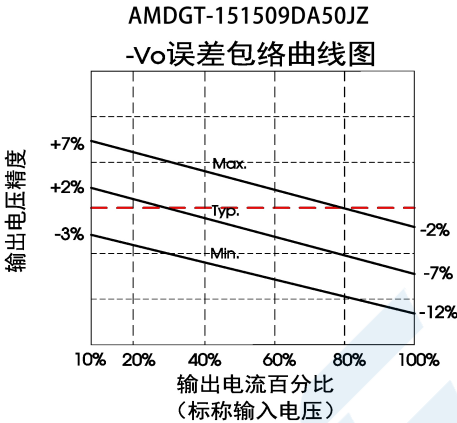
图 7 (辅路误差包络曲线)
