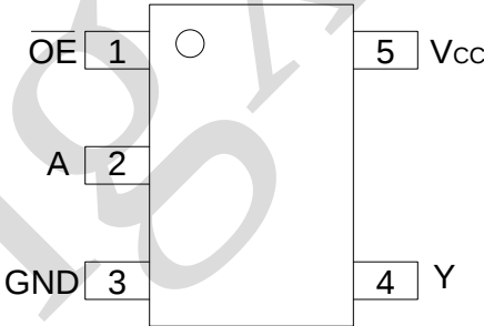
图 4 引脚排列图
