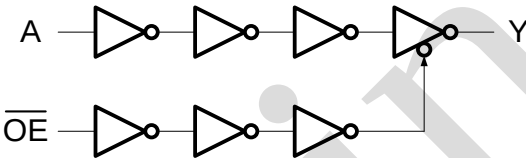
图 3 逻辑框图
