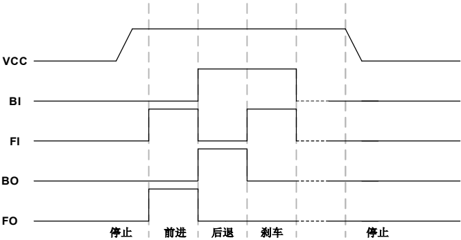
图 3. 输出时序图
