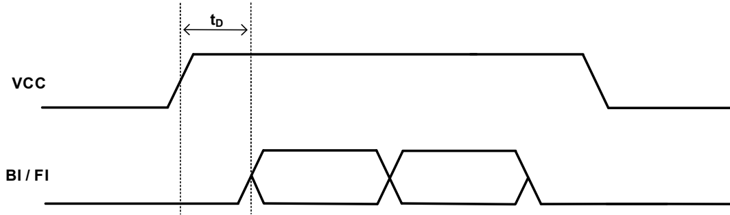
图 5. 上电时序图
