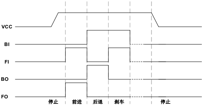
图 3. 输出时序图
