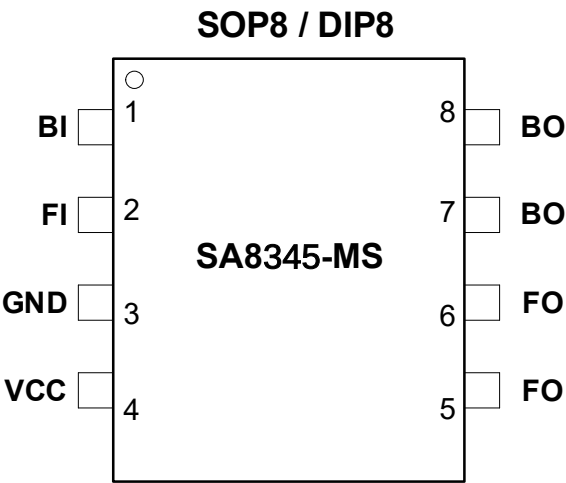
图 1. 顶视图
