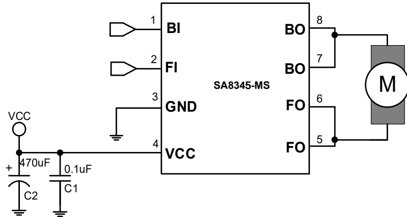
图 4. 应用原理图
