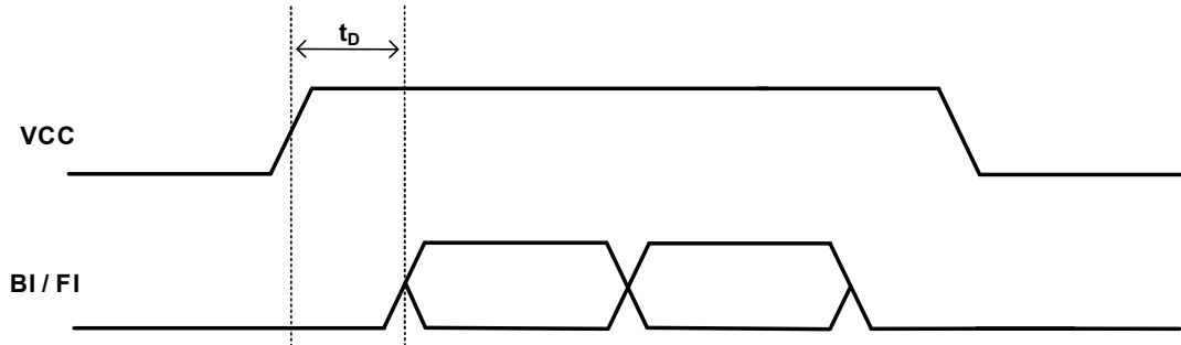
图 5. 上电时序图
