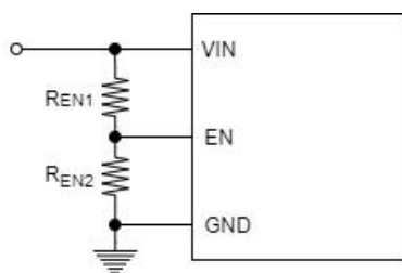
图1 欠压锁定分压电路
