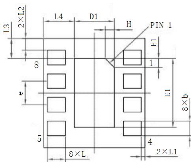
底视图
