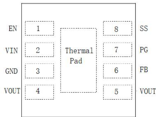
顶视图（透视）
