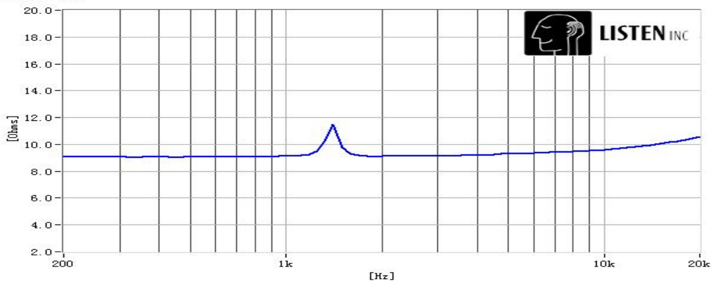
阻抗曲线
