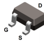
BSS123W SOT-323
