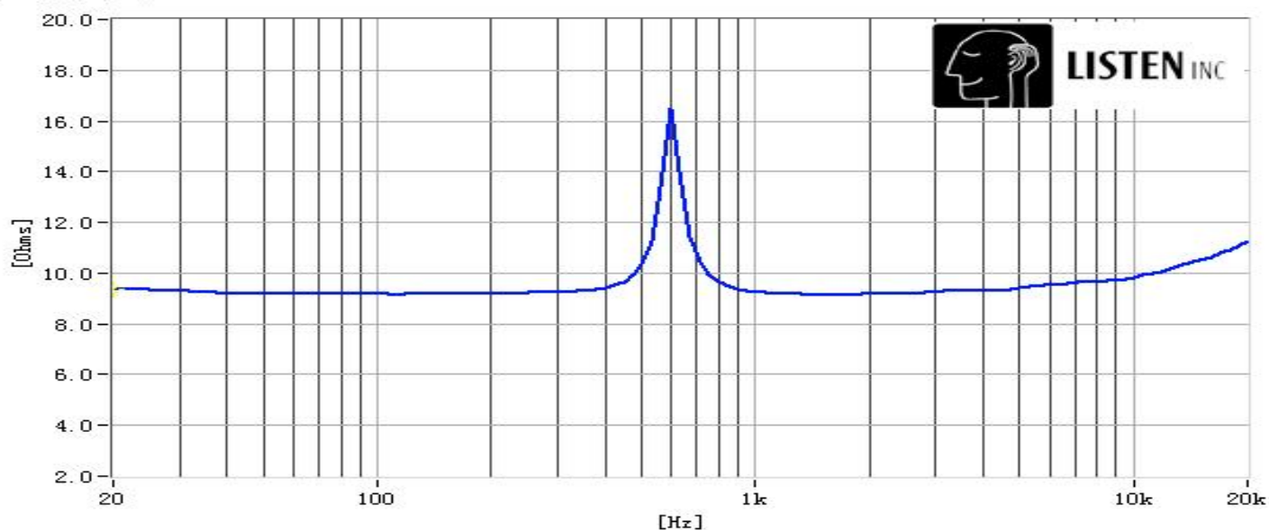
阻抗曲线
