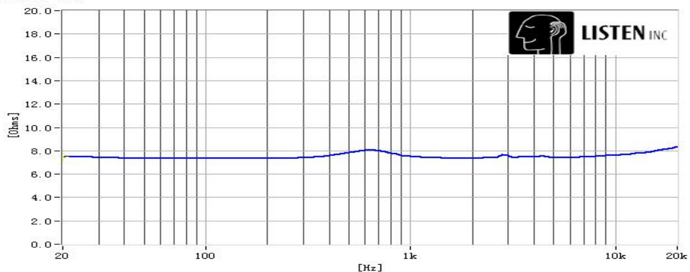
阻抗曲线
