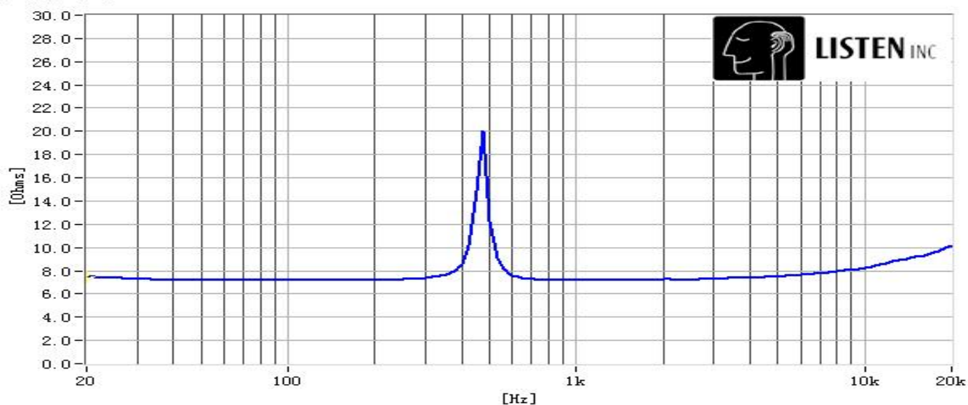
阻抗曲线
