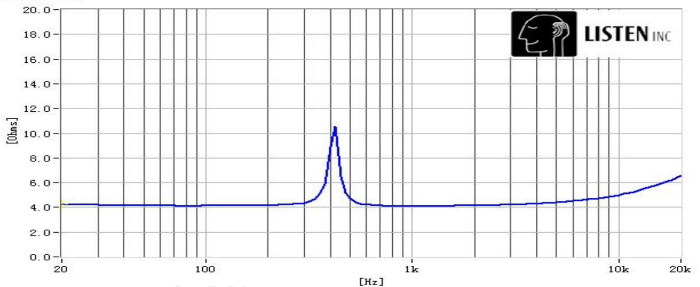
阻抗曲线
