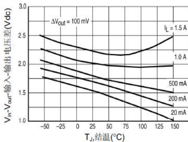
图 8. 压降电压
