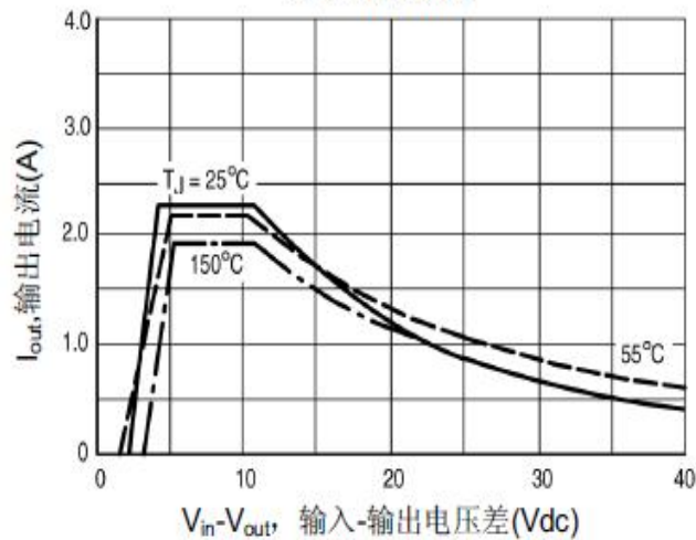
图 6. 电流限度
