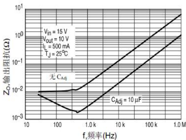
图 14. 输出阻抗
