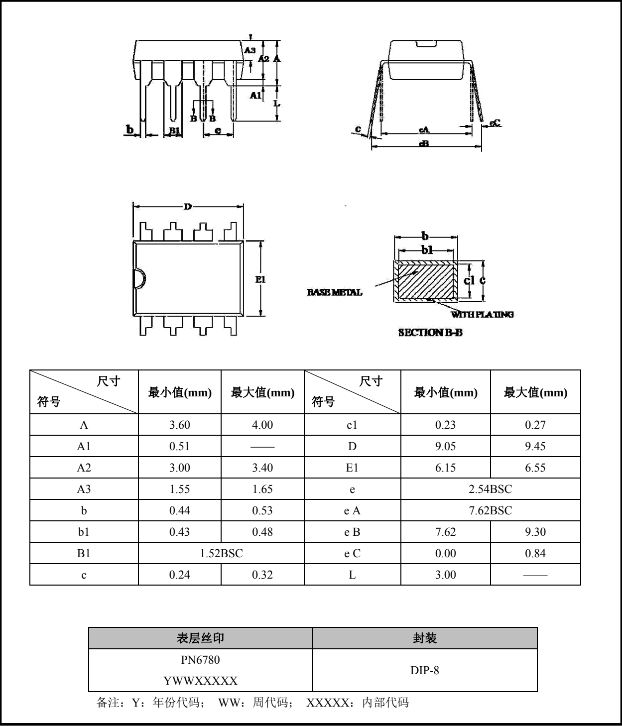
DIP-8 封装外形及尺寸
