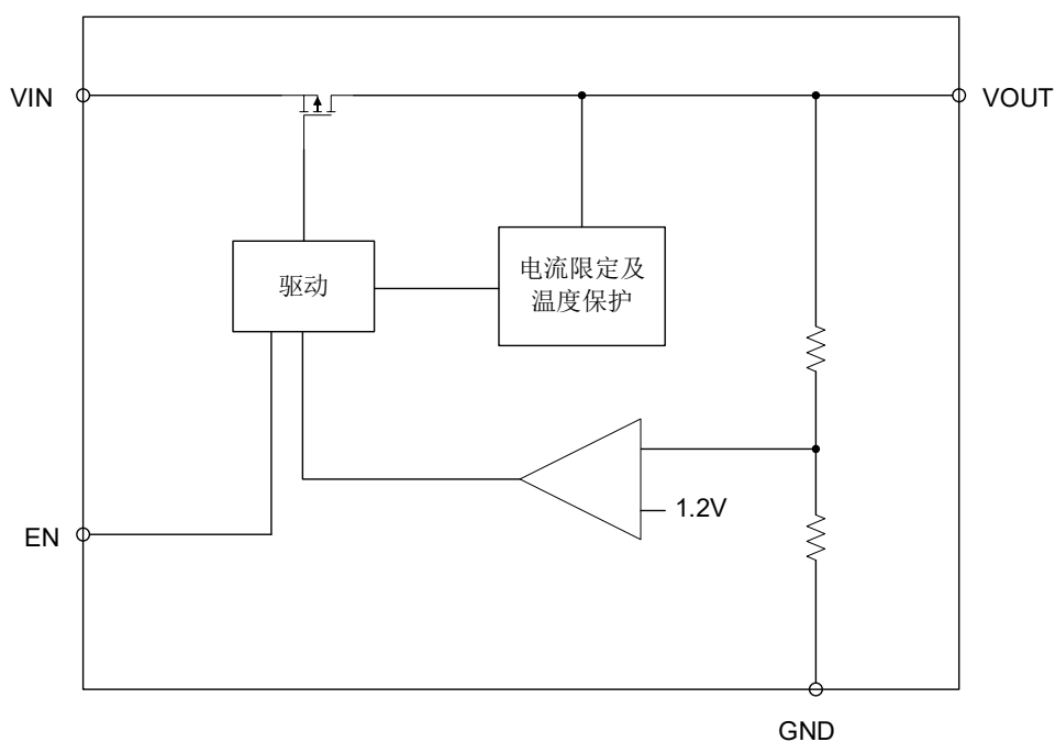
图 2 CM1843 系列 功能模块框图
