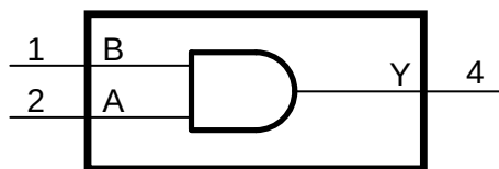
图 1 逻辑符号
