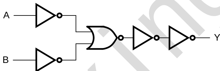
图 3 逻辑框图
