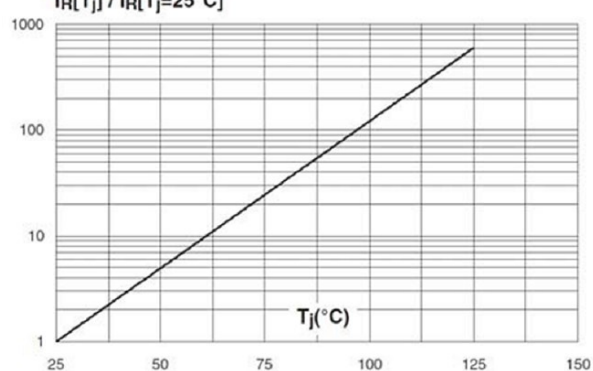
I_R(T_J) / I_R(T_J=25^\circ\text{C})
