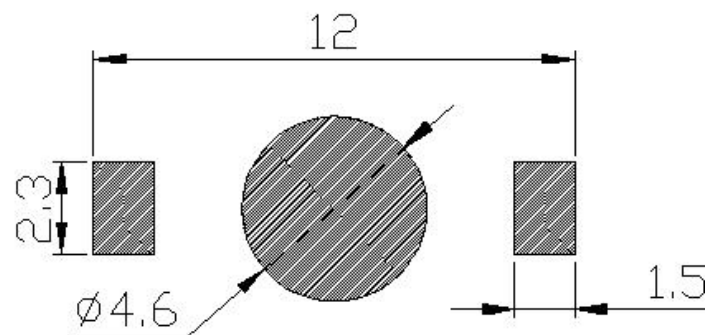
焊盘建议图
