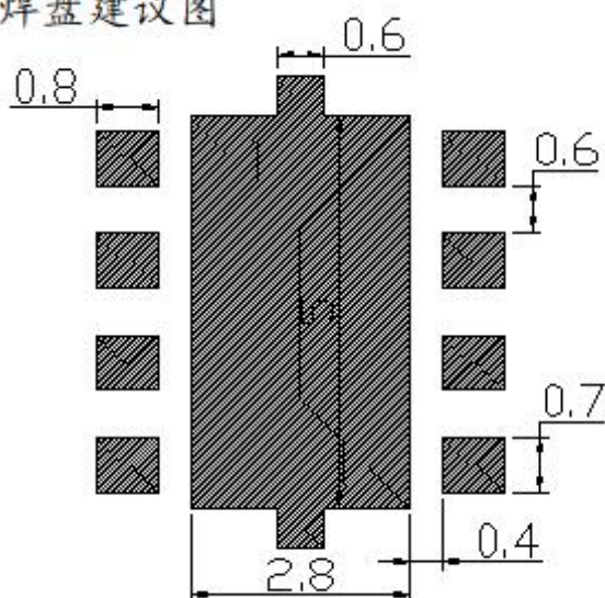
焊盘建议图
