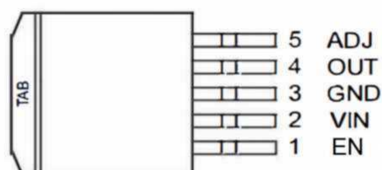
TO263
