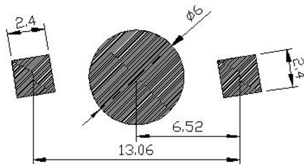
焊盘建议图
