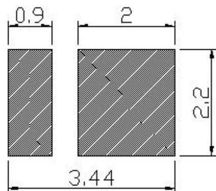
焊盘建议图
