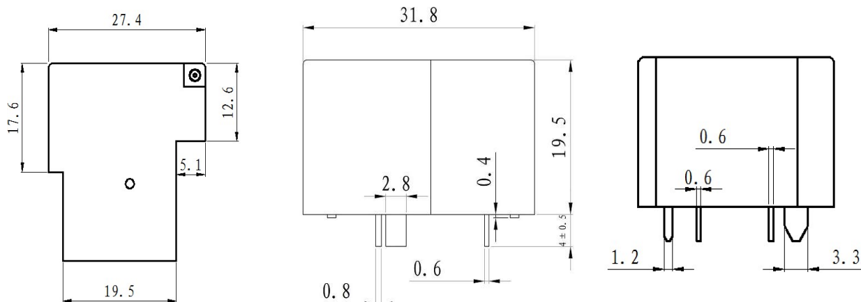
外形图 Layman
