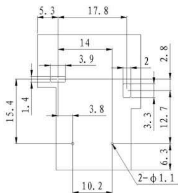
外形图 Layman
