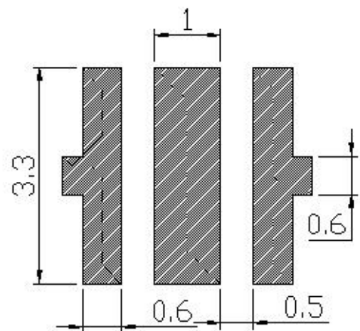
焊盘建议图
