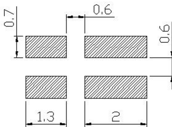
焊盘建议图
