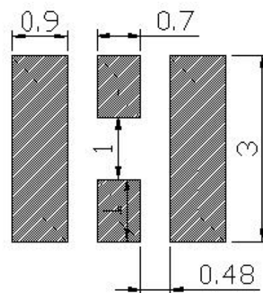
焊盘建议图
