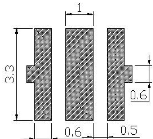
焊盘建议图
