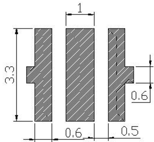
焊盘建议图
