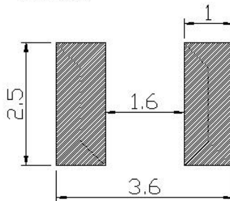
焊盘建议图
